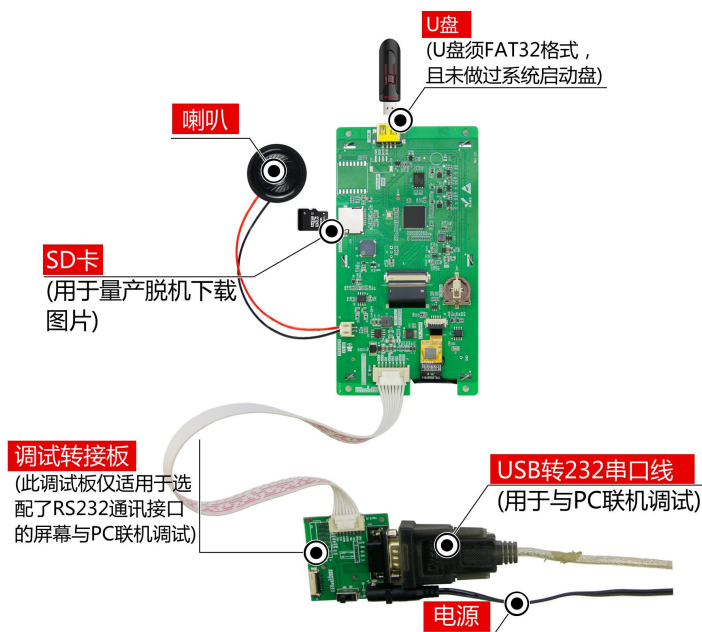
图 1-4 调试工具图
