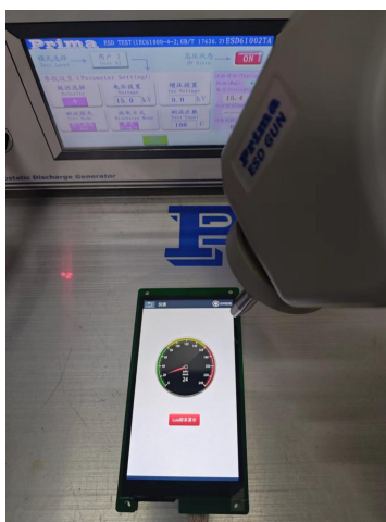
图 5-2 ESD 测试图
